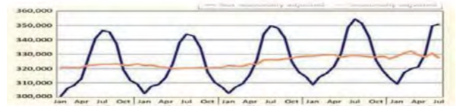
Grafik1: Mevsimsellikten arındırılmamış ve arındırılmış fark
